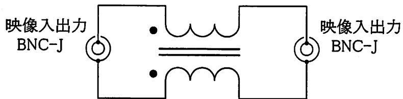
内部等価回路
